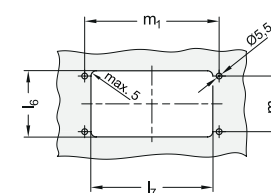
Montážní otvor
