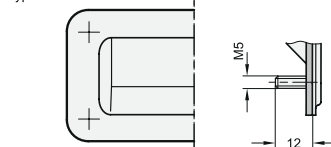
Montážní otvor
