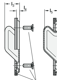
Zápuštěné těsnicí šrouby / Těsnění otvoru (pro označení č. 2)
